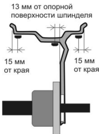
Рисунок 5.12 – Дистанции установки ленточных грузов
