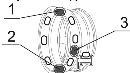
1 – груз в «12 час», 2 – груз в «6 час», 3 – установка груза линейкой
