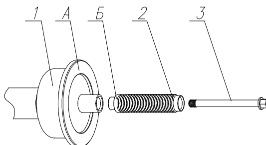
Рисунок 4.2 – Сборка вала
