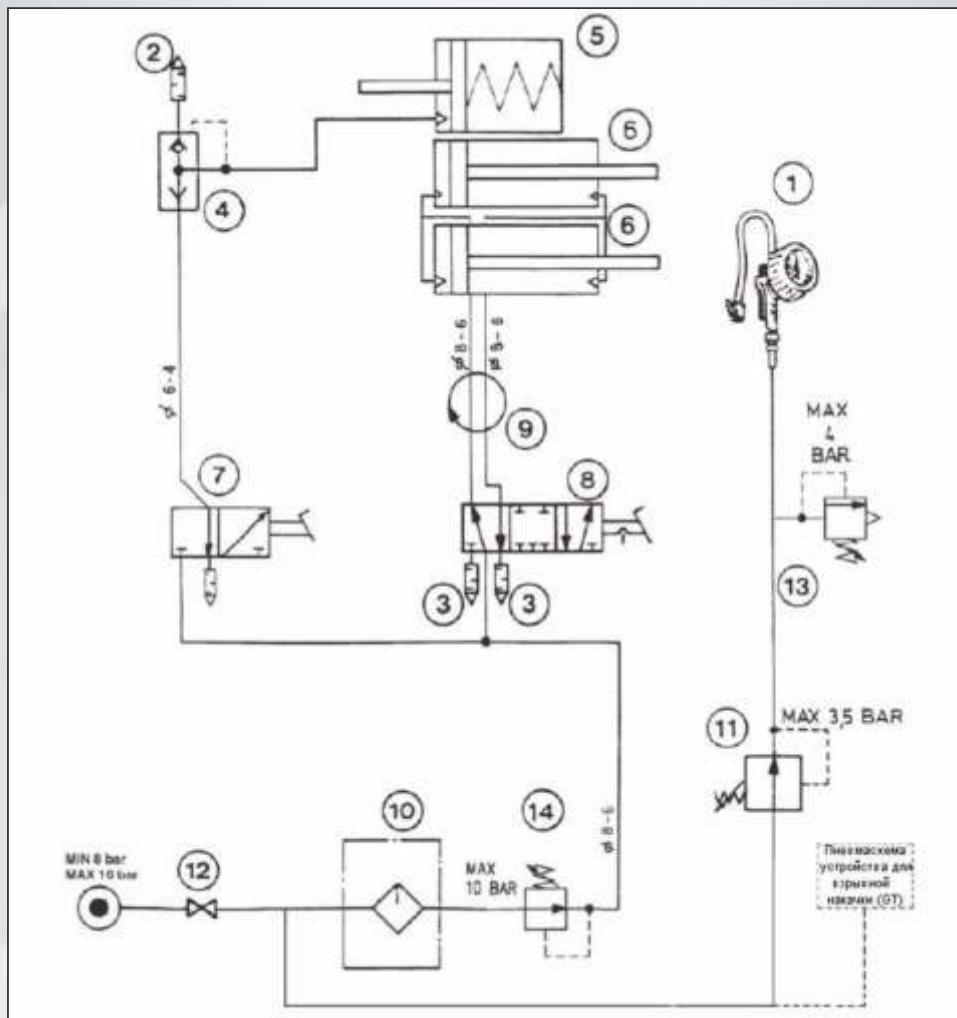
Пневматическая схема станда
